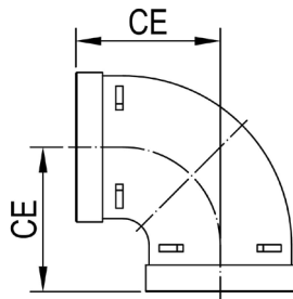
E1SS 90° Elbow
