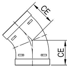
E2SS 45° Elbow
